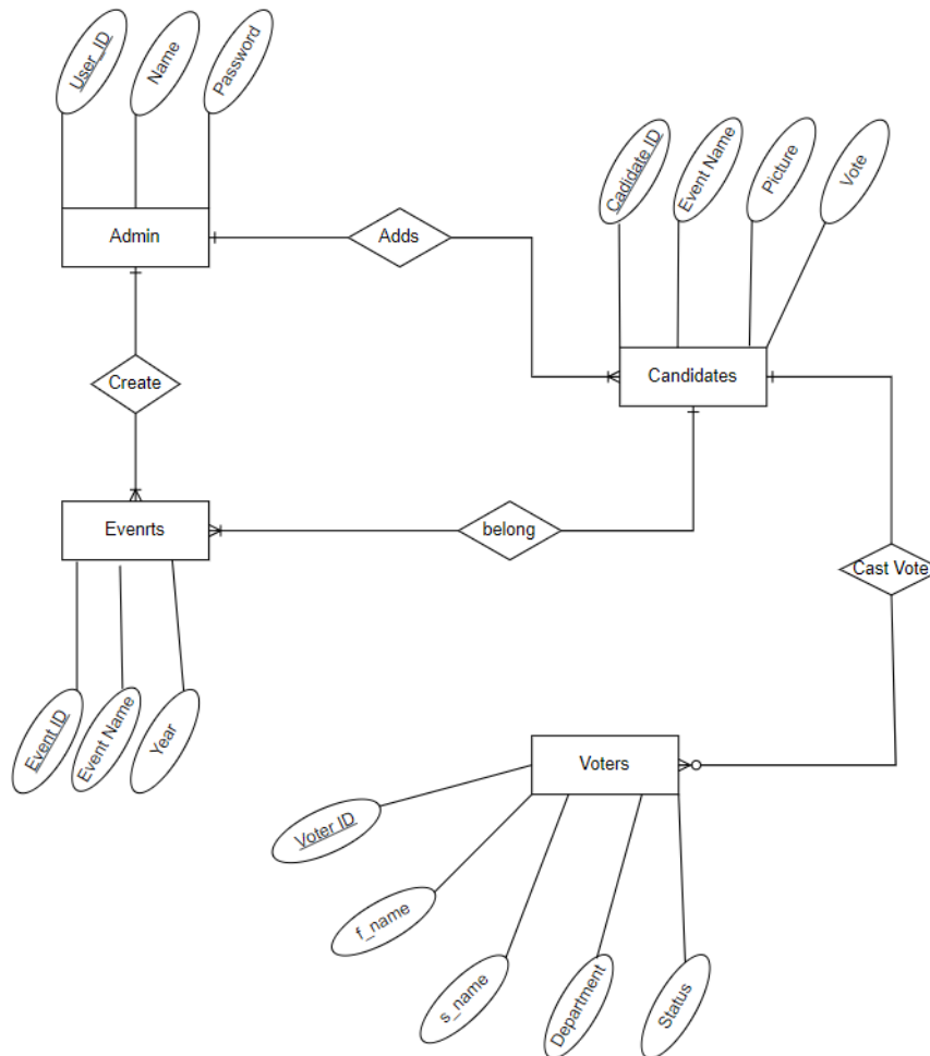
Figure 3: ER Diagram
